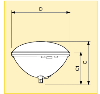
Boyutlar (mm)
