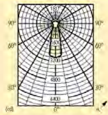
Işık dağılım eğrileri
